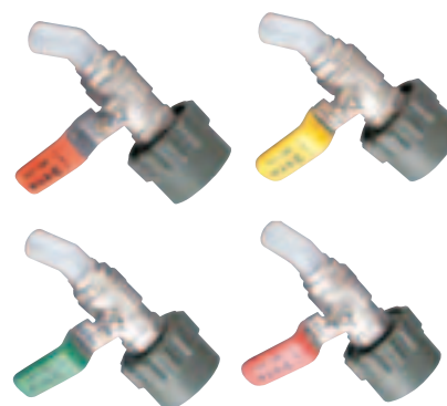
⑧ 一斗缶用バルブ MWC-40BS 〈KBL-41〉 目 ¥8,700 7-1456-0801 赤 7-1456-0802 緑 7-1456-0803 黄 7-1456-0804 オレンジ ●スカート (盛りあがり口) 外寸φ40mm専用。 ●ワンタッチ脱着で液こぼれがなくスムーズに注ぐことができます。 ●中身がわかり難い液体をレバーの色で区分けできます。
