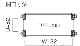
ステンレスポスト
